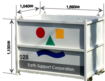
(外寸法)
